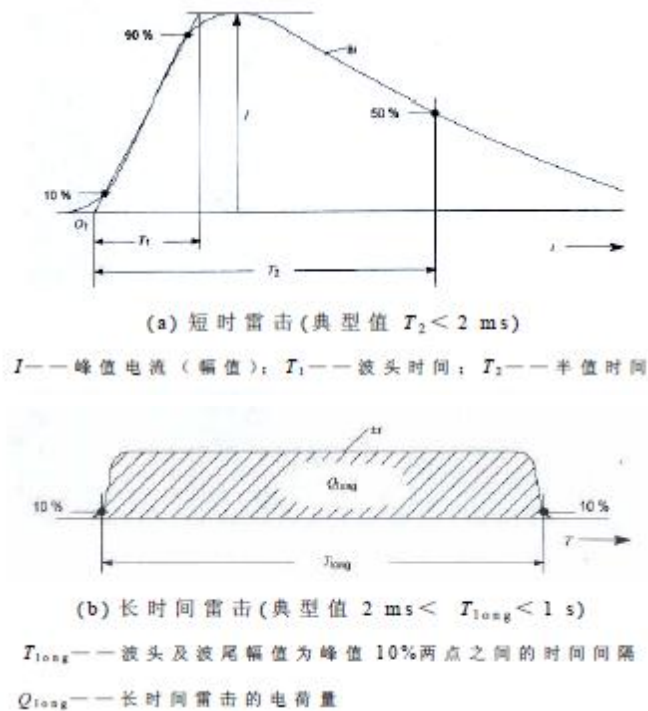
图 F.0.1-2 雷击参数定义
