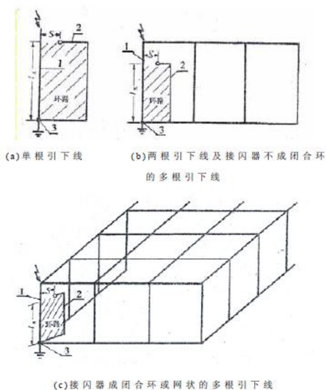
图 E.0.1 分流系数 k_c (1)
