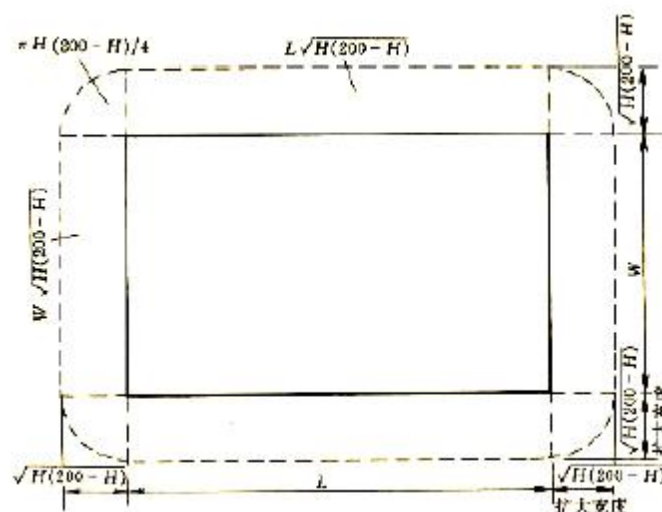
图 A.0.3 建筑物的等效面积
